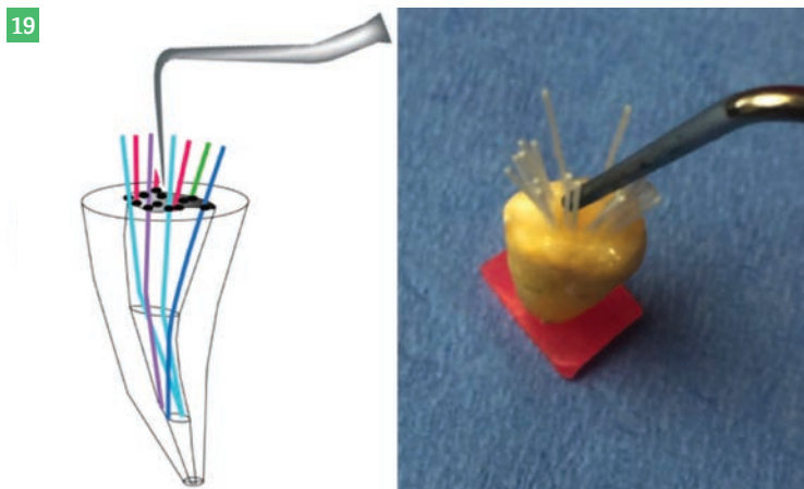
Fig.19 : Réorganisation des micro-tenons en privilégiant la périphérie.
