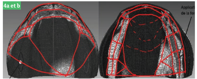
Fig.3a : Contraintes extrados. Fig.3b : Contraintes intrados. Fig.4a : Trajet théorique des renforts extrados. Fig.4b : Trajet théorique des renforts intrados. Fig.5a : Grille et tresse FiberForce. Fig.5b : Trajet compilé des renforts extrados + intrados. Fig.6: Structure d'une tresse hybride.
